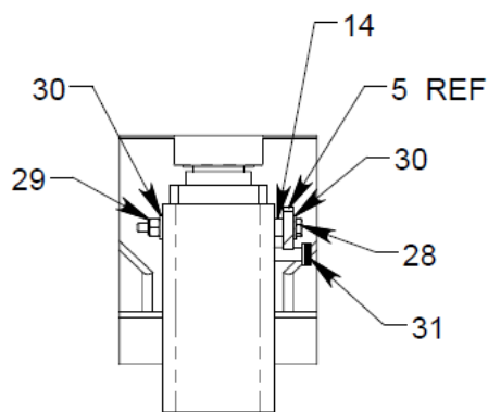
SECTION B-B SCALE 1 : 6
