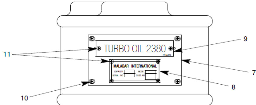
VIEW A-A
